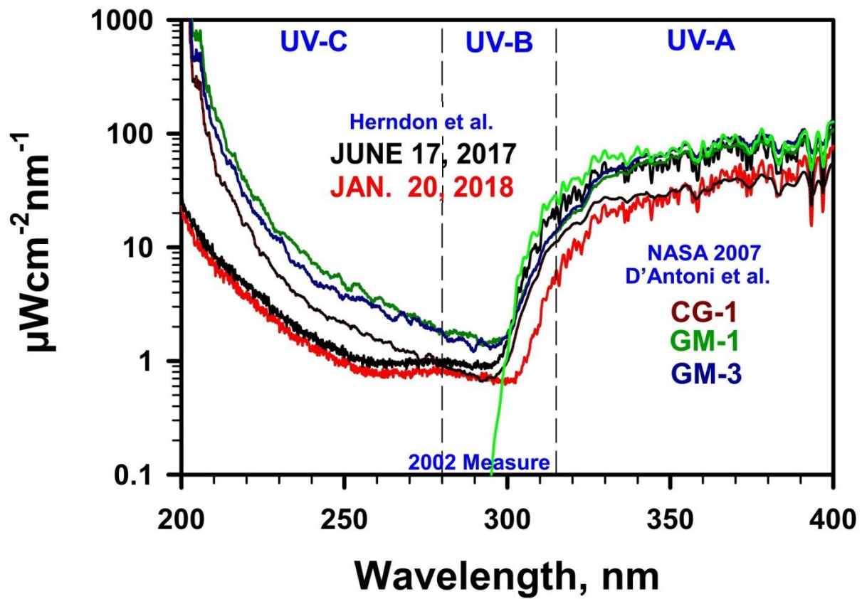
Figura 2: Mediciones solares espectrométricas. Observar las mediciones de 2002 que muestran el concepto común erróneo de no radiación UV-C en la superficie terrestre.
